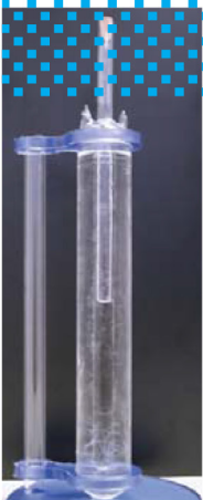
Celda del punto triple
