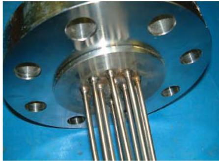
Brida de conexión multipunto
